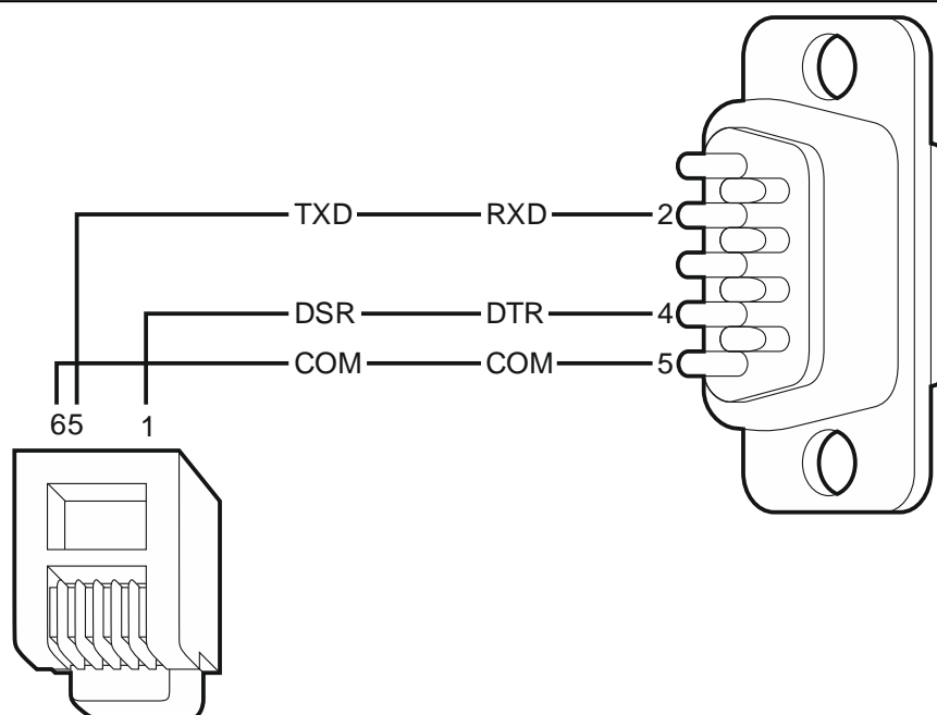
Rys. 15. Sposób podłączenia drukarki za pośrednictwem wtyku męskiego DB-9 (widok od strony punktów lutowniczych). Po lewej wtyk RJ podłączany do gniazda na płycie głównej centrali.
