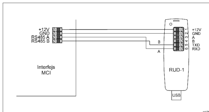
Rys. 2 Podłączenie interfejsu MCI-3 do RUD-1 w celu aktualizacji oprogramowania
